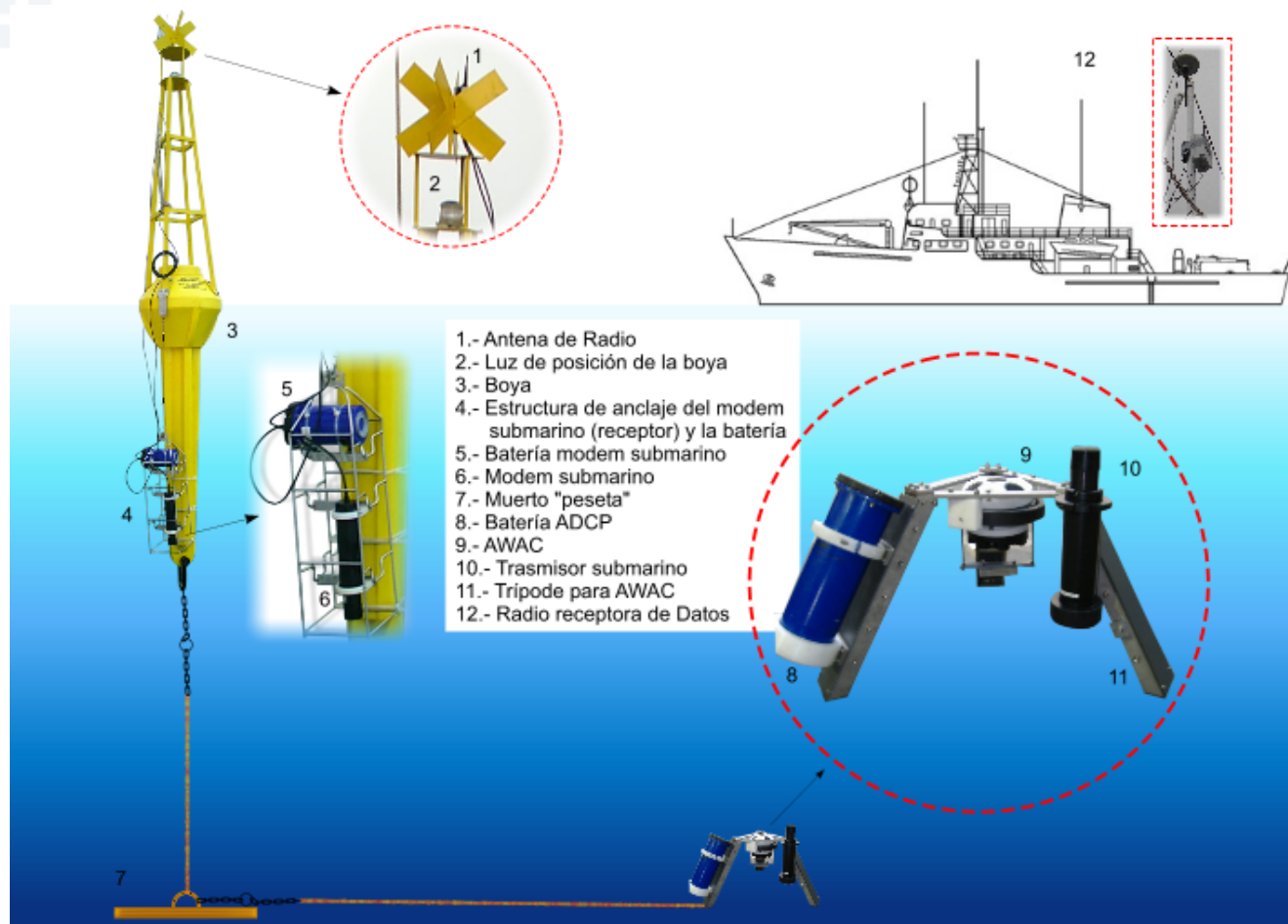
Sistema para obtención de corrientes y oleaje en tiempo real
